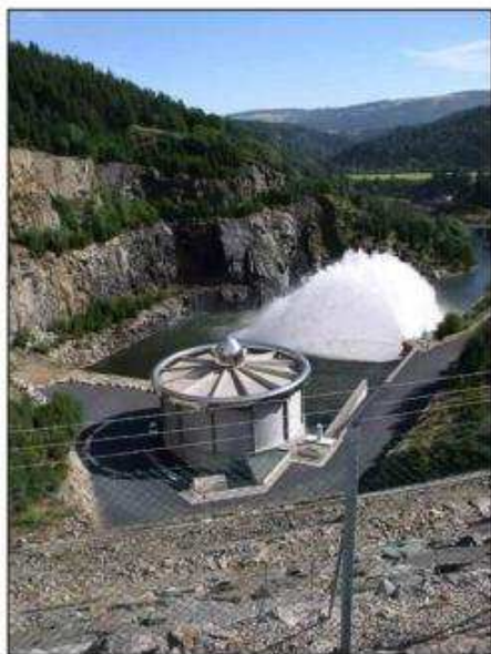
Le barrage de Naussac, en Haute-Loire. (Photo : Établissement public Loire)
